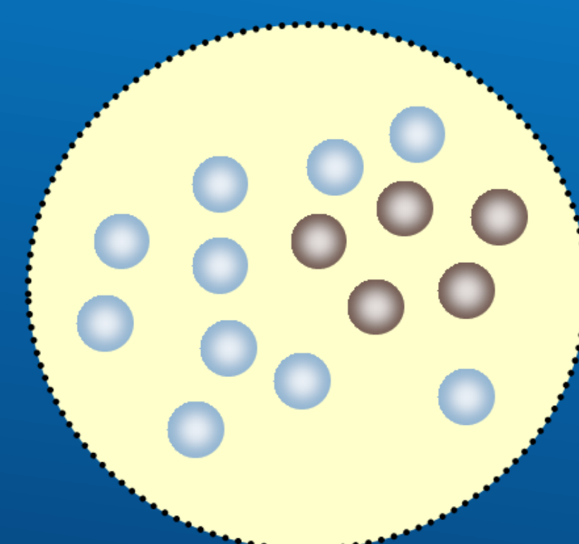
10 Mavi 5 Siyah
