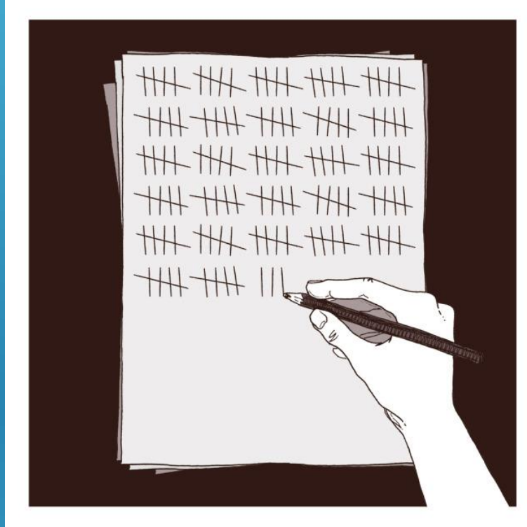
Abaküs - MÖ
