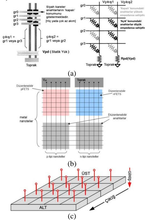
Şekil 2: Diyot tabanlı (a) [8], CMOS tabanlı (b) [9] ve dört-üçlü anahtar tabanlı nano-dizinler (c) [10].
