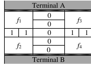
Şekil 8: f 1 = f 1 f 2 + f 3 f 4 fonksiyonunun nano-dizinler ile gerçekleştirilmesi.
