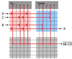
Şekil 5: f = (AB + CD) fonksiyonunun CMOS tabanlı nano-dizinler ile tasarımı [9].
