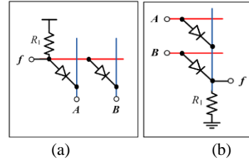
Şekil 3: f = AB (a) ve f = A + B (b) fonksiyonlarının diyot tabanlı nano-dizin tasarımları.
