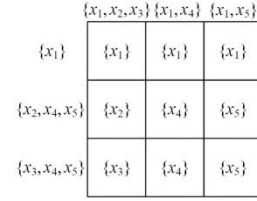
Şekil 5: f = x_1x_2x_3 + x_1x_4 + x_1x_5 fonksiyonunun dört-üçlü anahtar tabanlı nano-dizinler ile tasarımı [10].
