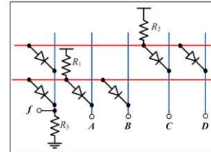
Şekil 4: f = AB + CD fonksiyonunun diyot tabanlı nano-dizinler ile tasarımı.
